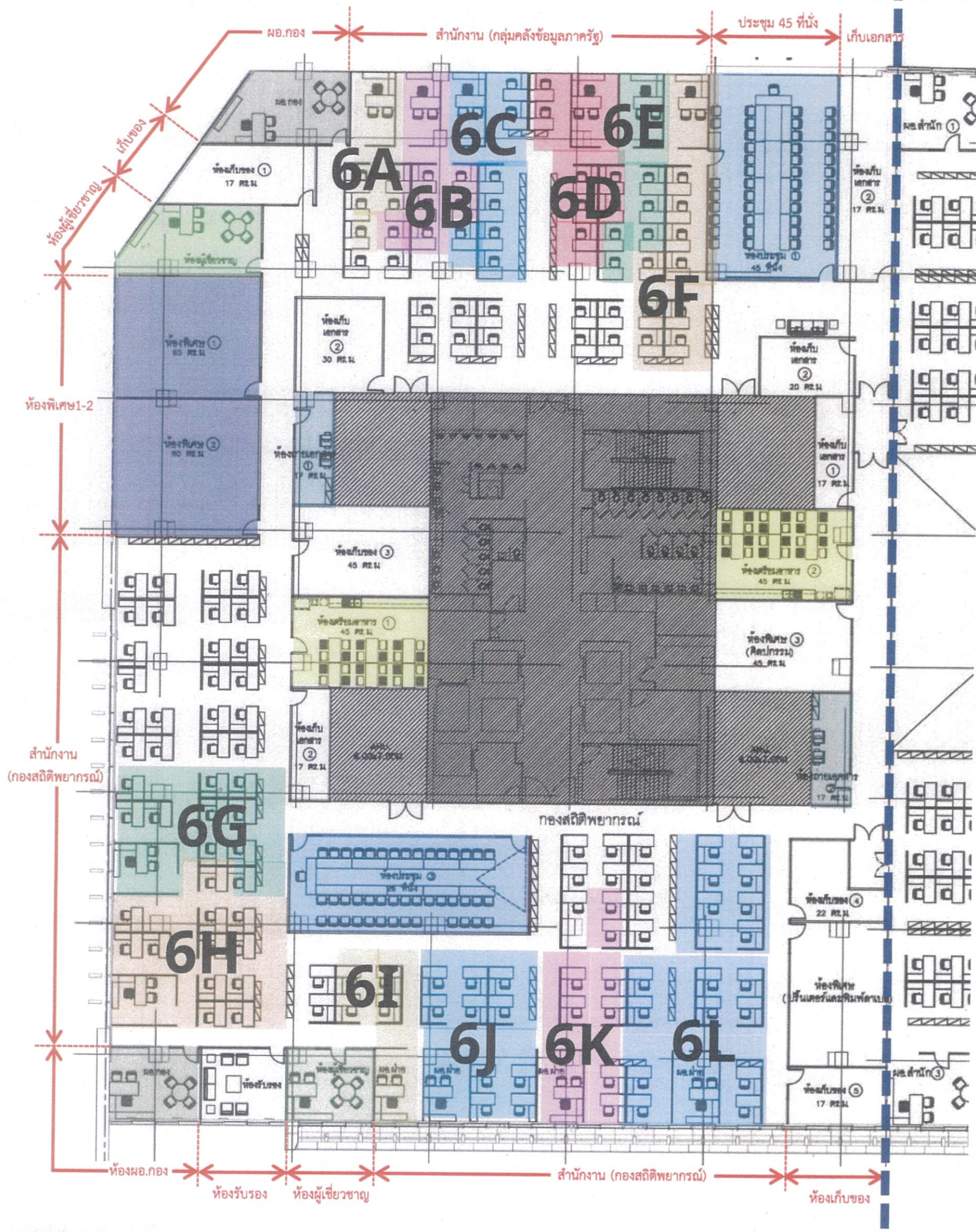
แปลนพื้นที่ชั้น 6
